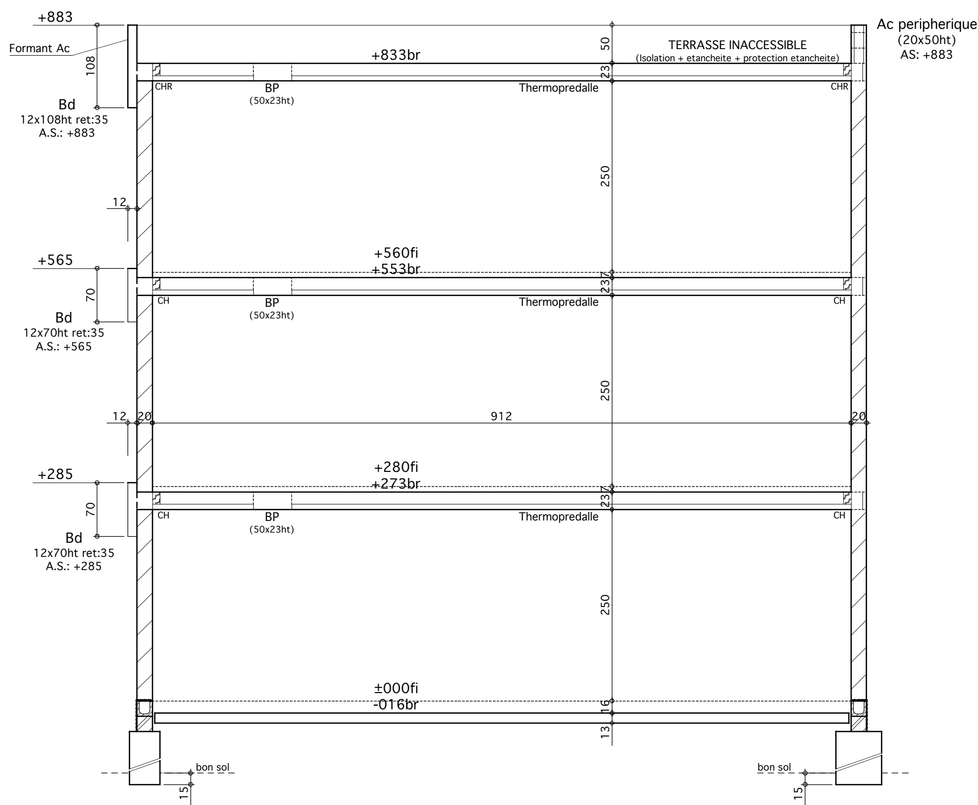
COUPE 1.1
