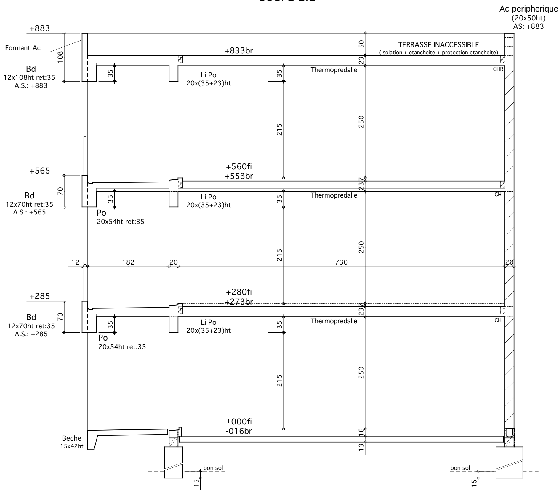
COUPE 2.2
